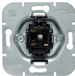
Moduł łącznika
