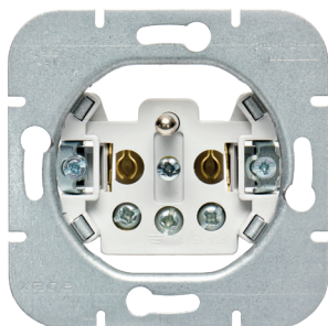
Moduł gniazda
